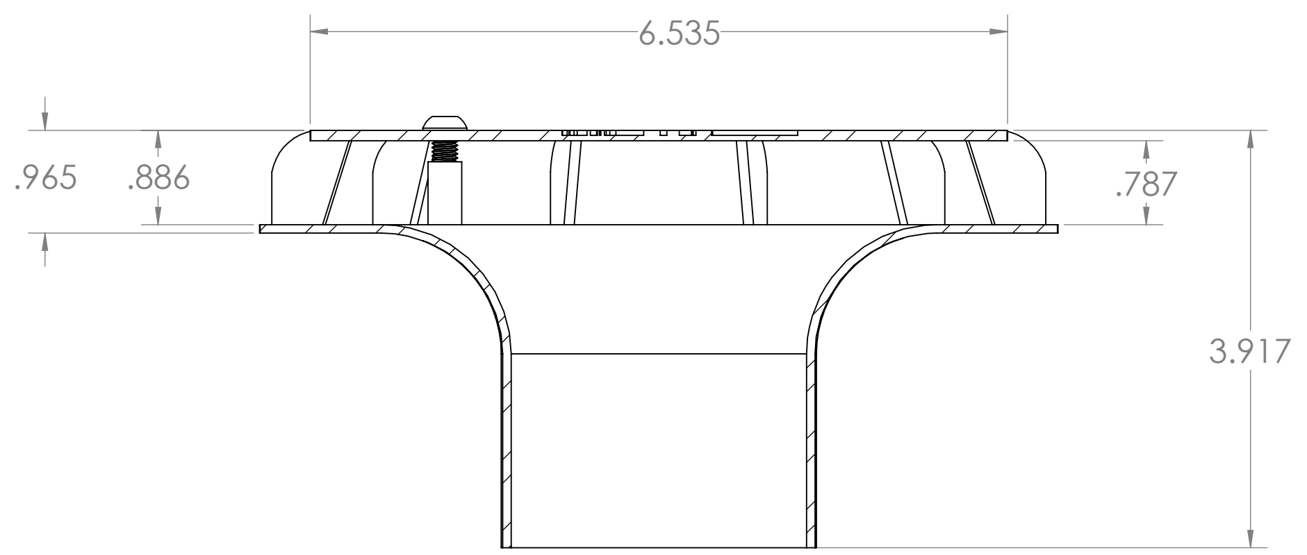
SECTION A-A SCALE 1 : 1.25
